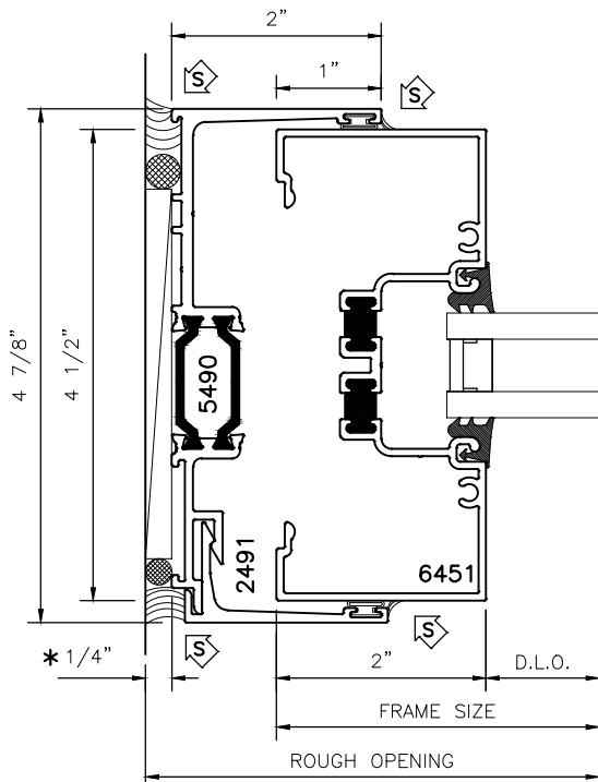
LEFT JAMB
