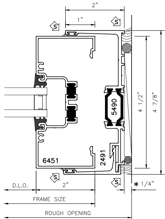
RIGHT JAMB
