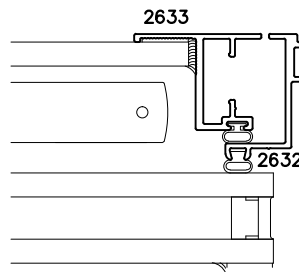
RIGHT JAMB
