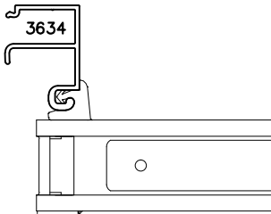
LEFT JAMB
