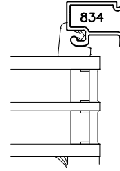
RIGHT JAMB
