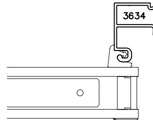
RIGHT JAMB
